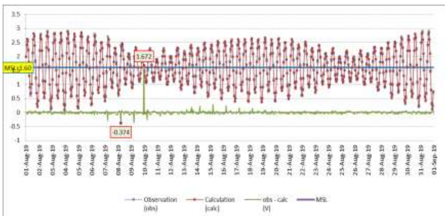
Grafik 9. Tinggi Muka Air Pasang Surut, Tanjung Tiram, Batu Bara
