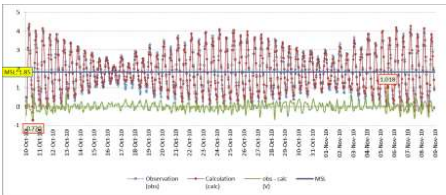
Grafik 10. Tinggi Muka Air Pasang Surut, Panai, Labuhan Batu
