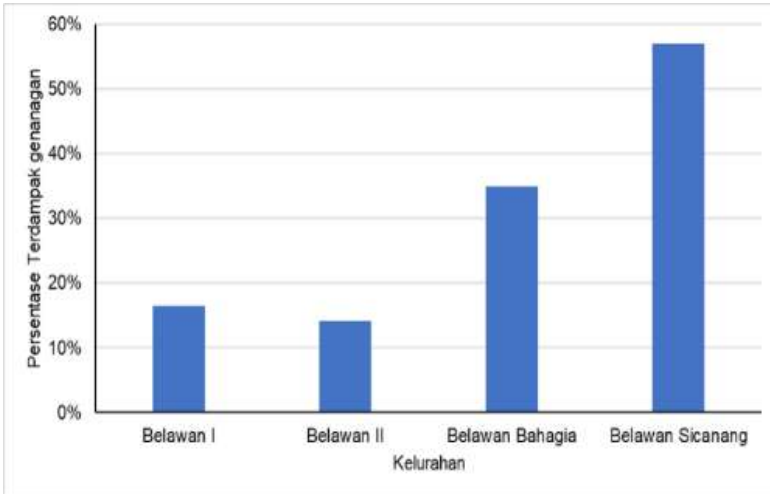
Grafik 11. Kerentanan Bencana Banjir dan Rob di Belawan. A. Persentase Luas Kawasan Terdampak per Kelurahan
