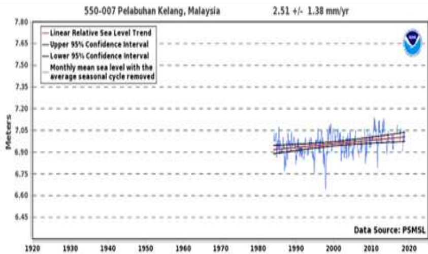
Grafik 5. Kenaikan Muka Air Laut – Pelabuhan Kelang, Malaysia
