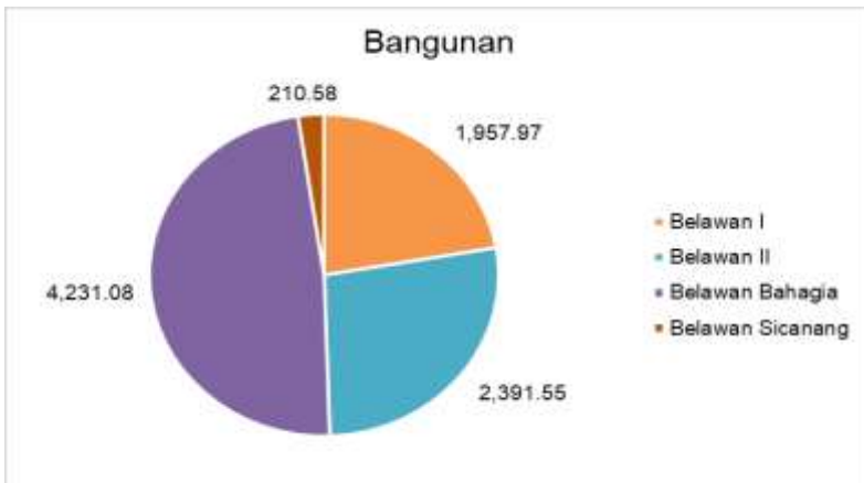
Grafik 14. Kawasan Bangunan Mengalami Dampak Akibat Air Pasang di Belawan
