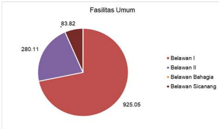
Grafik 13. Kawasan Fasilitas Umum Mengalami Dampak Akibat Air Pasang di Belawan
